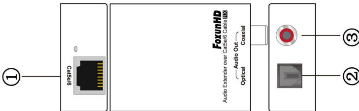
AEX01-RX 正面面板
